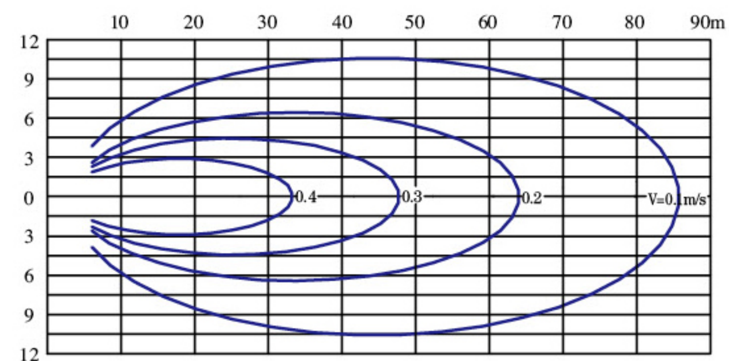
QDTA1800/47/2-5.5/G QDTA2100/47/2-5.5/G
