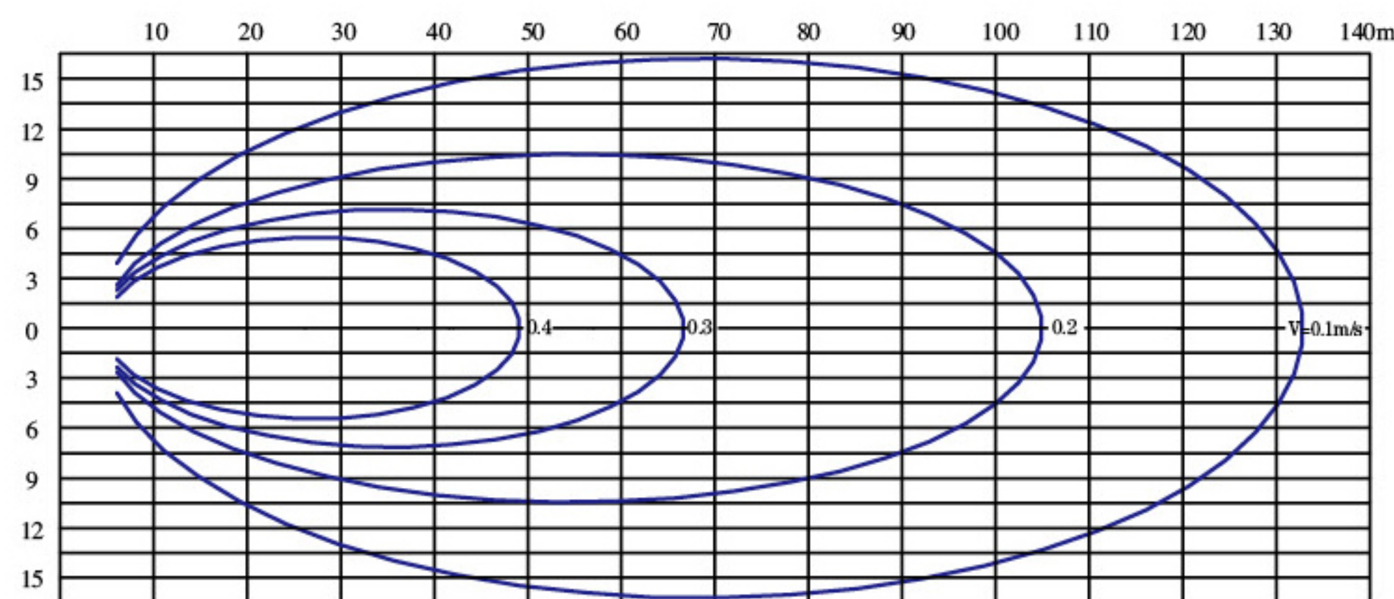
QDTA2500/43/3-7.5/G
