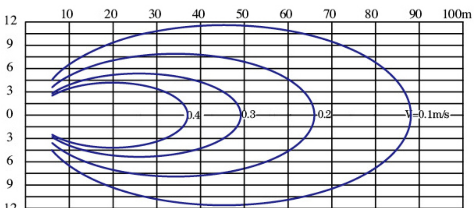
QDTA2100/43/3-5.5/G
